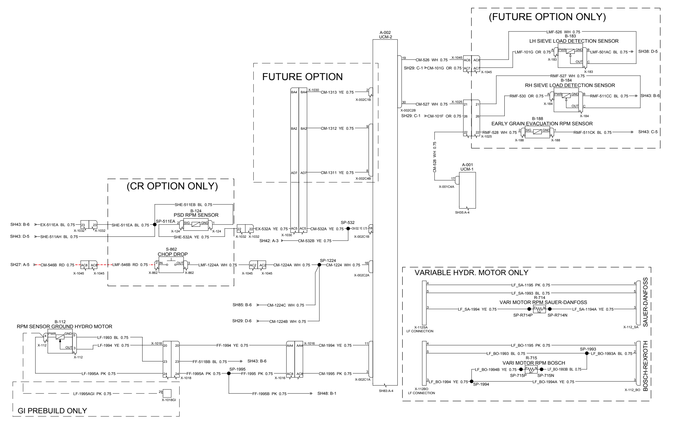
SHEET 44 - UCM2-VARIABLE MOTOR & FAN
