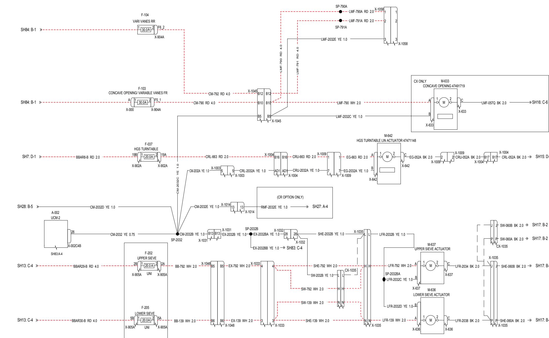
SHEET 30 - SIEVE LIN & CONCAVE ACTUATOR
